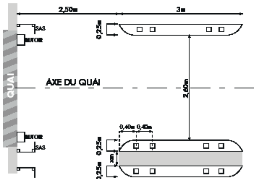
PLAN D'IMPLANTATION
